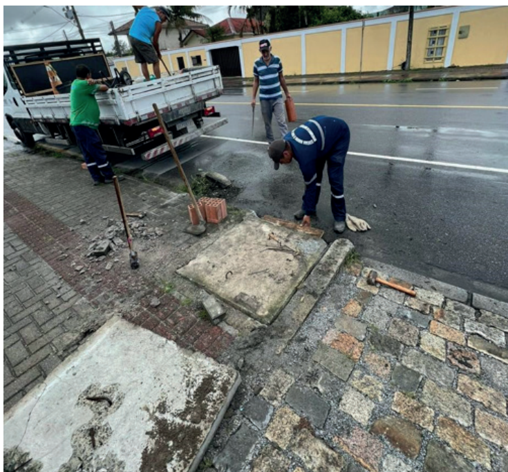
17. Manutenção em boca de lobo na Av. Belmiro Sebastião Marques – Parque São João
